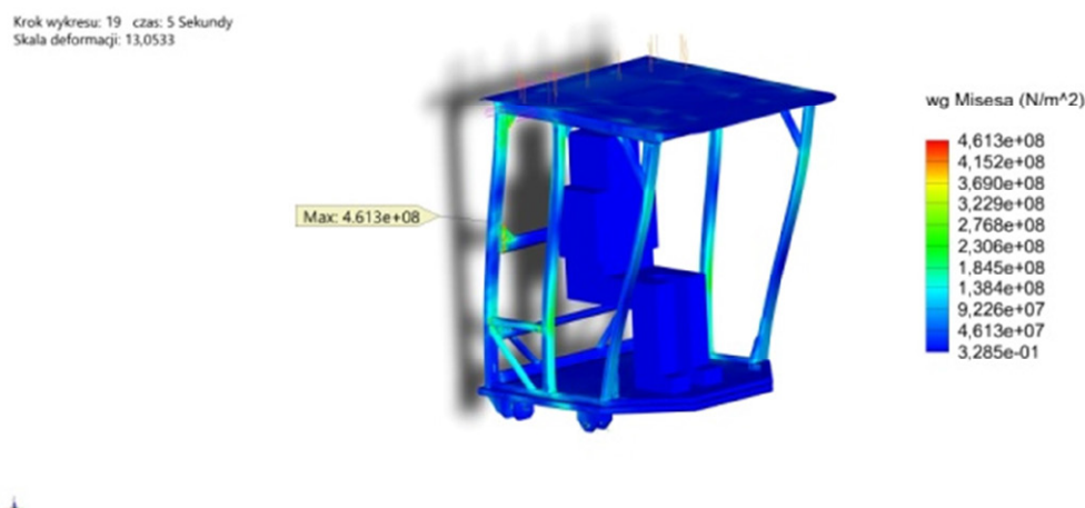
Fig. 17. Stress distribution (von Mises)
