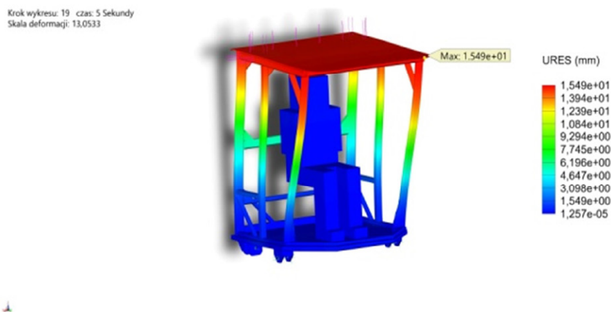
Fig. 18. Displacement distribution
